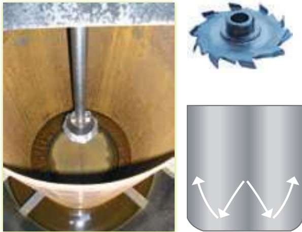
Figure 14. Mélangeur à disque Cowles
